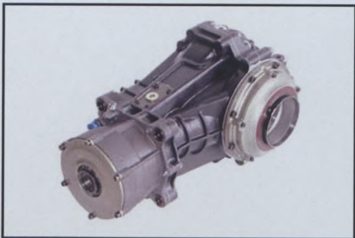
DI3-3) Carter du différentiel (vue 1) Differential housing (view 1) :
