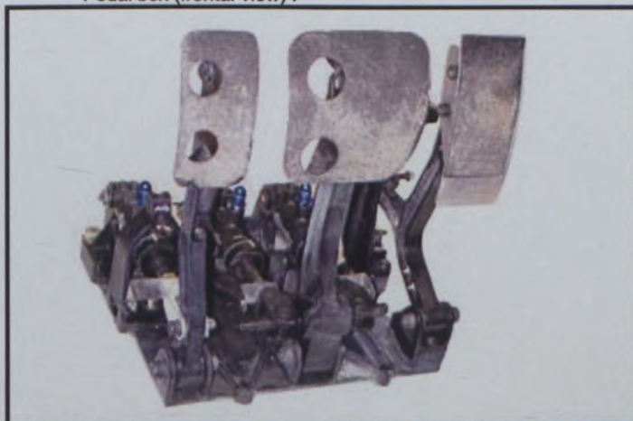
PED1) Pédalier (vue de face) : Pedal box (frontal view) :
