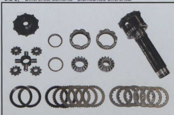
DI2-2) Différentiel démonté - Dismounted differential
