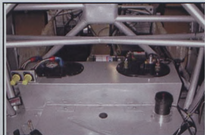
RE4) Réservoir à essence monté (vue de l'habitacle) Fuel tank mounted (seen from the cockpit)
