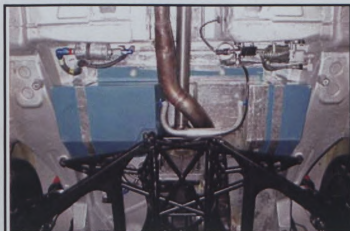
RE3) Réservoir à essence monté (vue de dessous) Fuel tank mounted (seen underneath)
