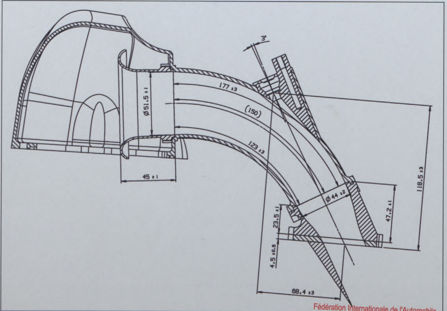
I3) Collecteur d'admission (dessin) Intake manifold (drawing)
