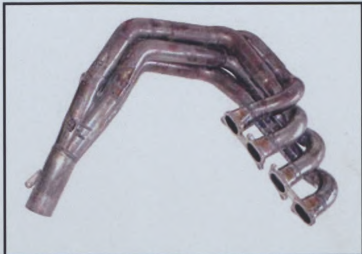
J1) Collecteur d'échappement (photo n°1) Exhaust manifold (photo n°1)
