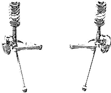
Photo E 車から 取外した完全なリアサスペンションアッセンブリー(ホイールを除く) Complete rear wheels assy removed from car. (without wheels).
