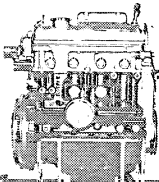
Photo I エンジン右側面(エンジン補器、マニホールド、インテーク、ファンを取外す。 View of the engine, right side, without accessories, without manifold(s) intake nor fan.
