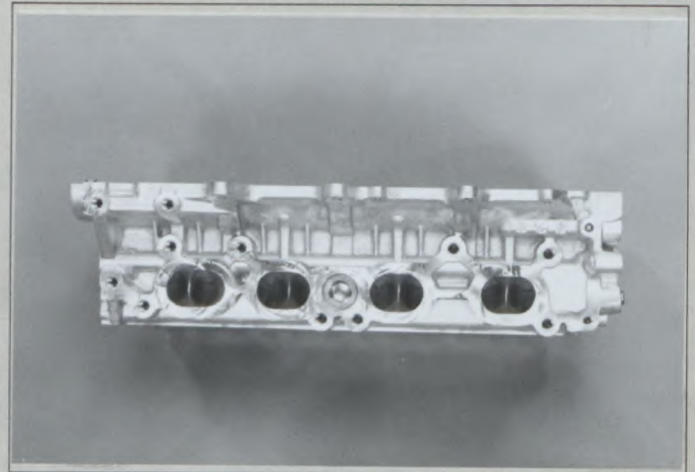
F2) Profil gauche de culasse nue Left hand view of bare cylinderhead シリンダーヘッド単体の左面
