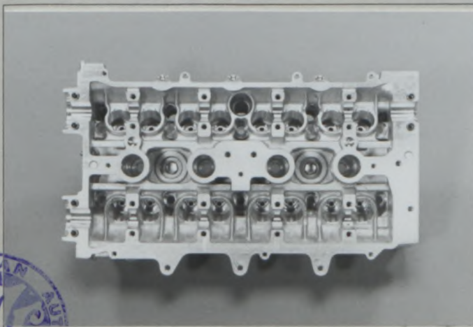
F1) Culasse nue vue de dessus Bare cylinderhead seen from above シリンダーヘッド単体の上面
