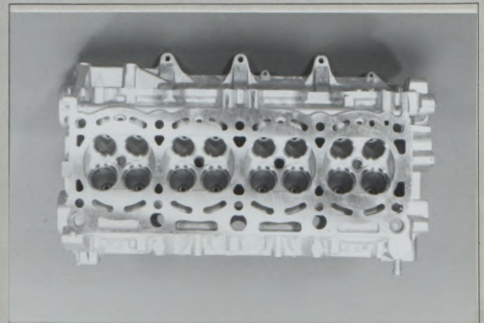
F2) Culasse nue vue de dessous Bare cylinderhead seen from below シリンダーヘッド単体の下面
