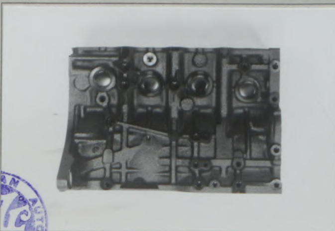
C3) Profil droit du bloc nu Right hand view of bare block ブロック単体の右面
