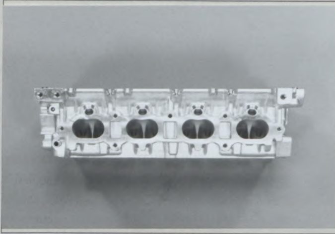
F1) Profil droit de culasse nue Right hand view of bare cylinderhead シリンダーヘッド単体の右面
