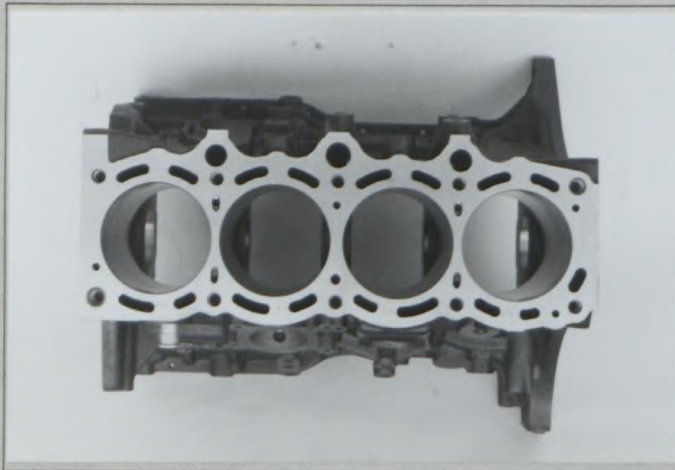
C1) Bloc nu vu de dessus Bare block seen from above ブロック単体の上面
