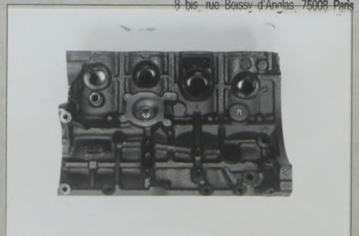
C4) Profil gauche du bloc nu Left hand view of bare block ブロック単体の左面
