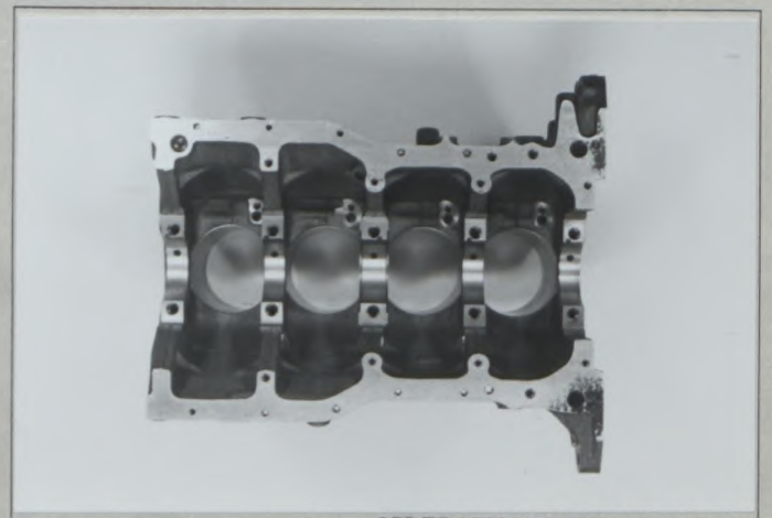
C2) Bloc nu vu de dessous Bare block seen from below ブロック単体の下面
