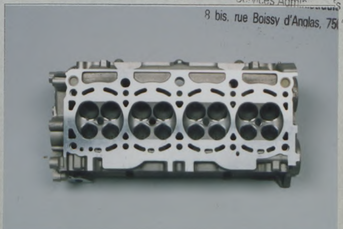
F2) Culasse nue vue de dessous Bare cylinderhead seen from below シリンダーヘッド単体の下面視
