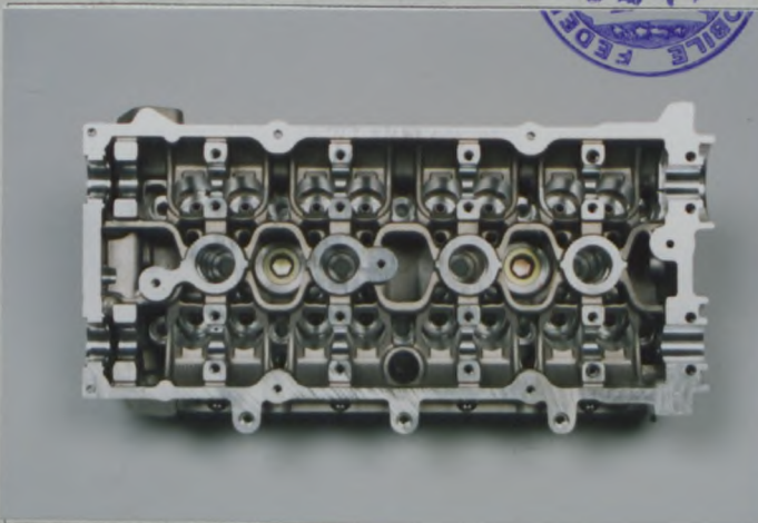
F1) Culasse nue vue de dessus Bare cylinderhead seen from above シリンダーヘッド単体の上面視
