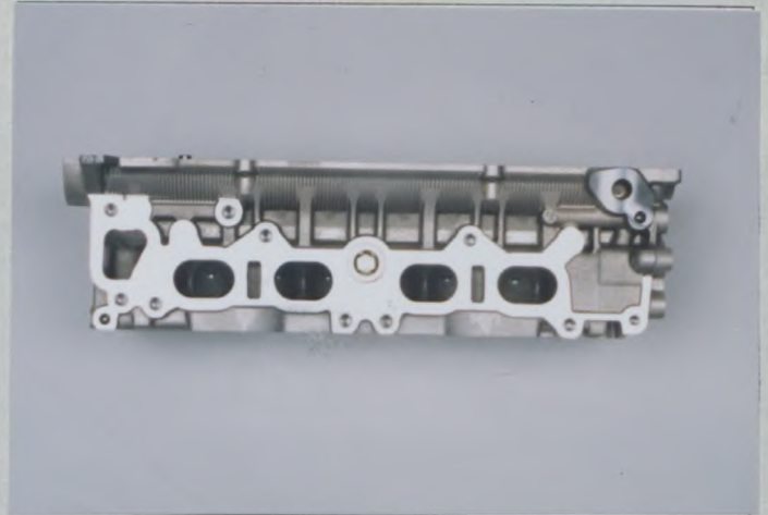
F2) Profil gauche de culasse nue Left hand view of bare cylinderhead シリンダーヘッド単体の左面視
