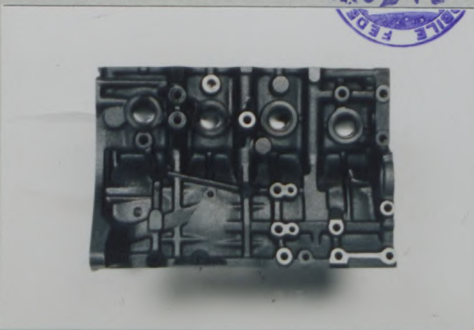
C3) Profil droit du bloc nu Right hand view of bare block ブロック単体の右面視
