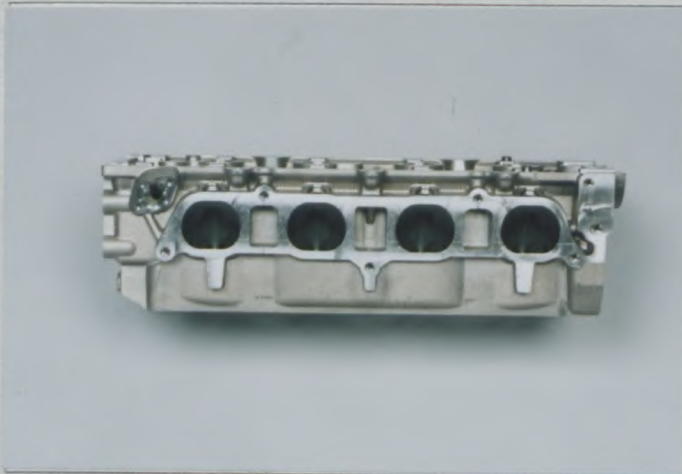
F1) Profil droit de culasse nue Right hand view of bare cylinderhead シリンダーヘッド単体の右面視
