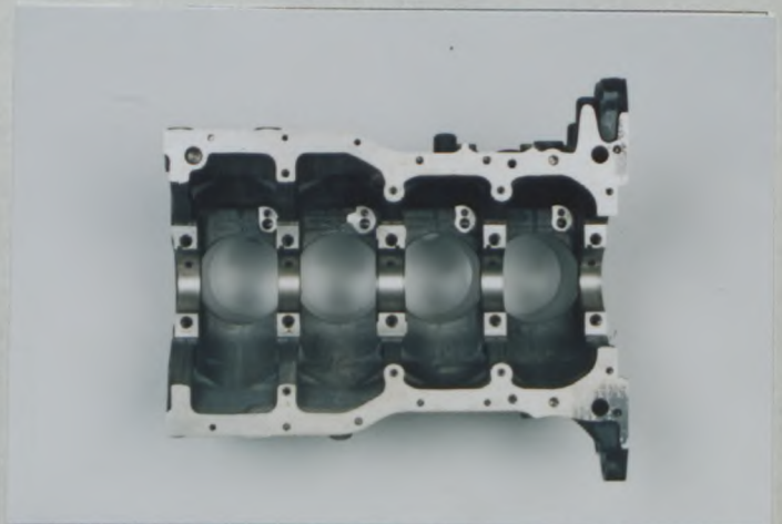
C2) Bloc nu vu de dessous Bare block seen from below ブロック単体の下面視
