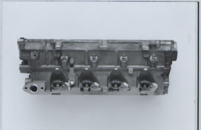
Profil gauche de culasse nue Left hand view of bare cylinderhead シリンダ'ヘッド'単体の左面視
