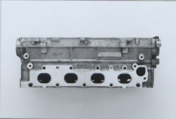
Profil droit de culasse nue Right hand view of bare cylinderhead シリンダ'ヘッド'単体の右面視
