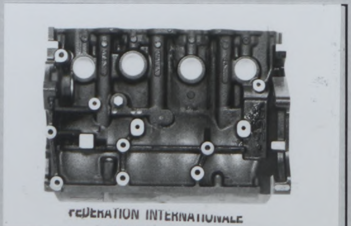
Profil gauche du bloc nu Left hand view of bare block ブロック単体の左面視
