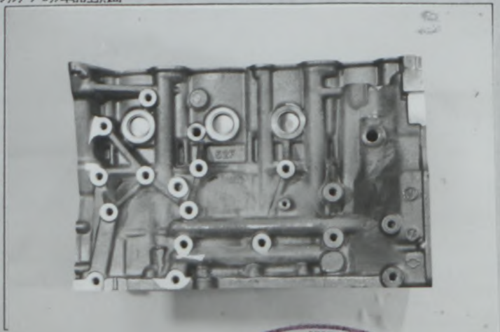
Profil gauche du bloc nu Left hand view of bare block シリンダーブロック単品左側面
