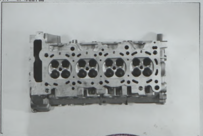
Culasse nue vue de dessous Bare cylinder head seen from below シリンダーヘッド 単品下面
