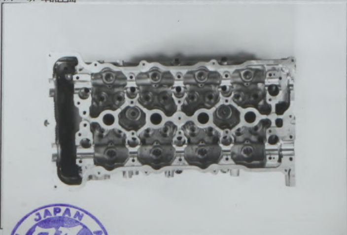
Culasse nue vue de dessus Bare cylinder head seen from above シリンダーヘッド 単品上面
