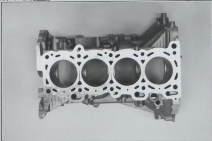
Bloc nu vu de dessus Bare block seen from above シタノット 単品上面
