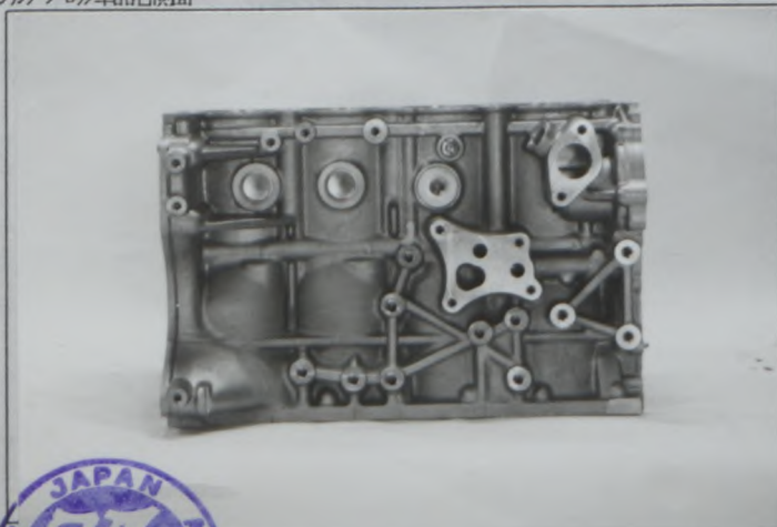
Profil droit du bloc nu Right hand view of bare block シタノット 単品右側面
