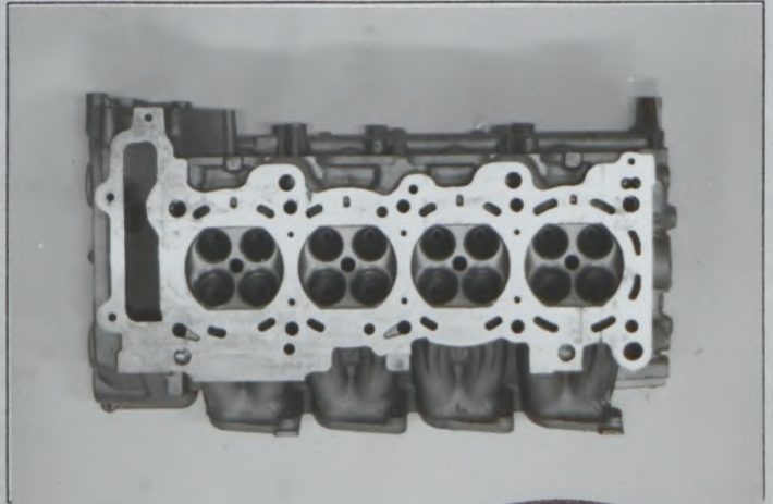
Culasse nue vue de dessous Bare cylinder head seen from below シリンダーヘッド 単品下面
