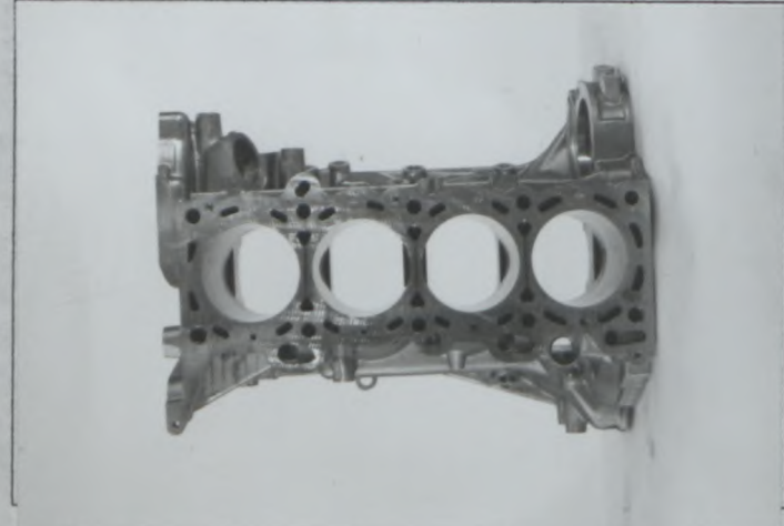
Profil droit du bloc nu Right hand view of bare block シリンダブロック単品右側面
