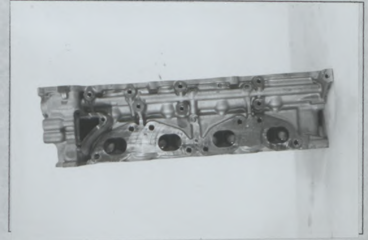
Bloc nu vu de dessous Bare block seen from below シリンダブロック単品下面
