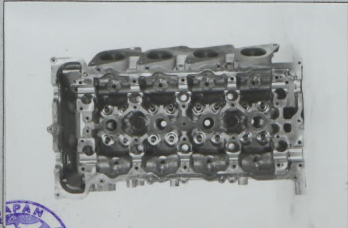
Culasse nue vue de dessus Bare cylinder head seen from above シリンダヘッド 単品上面
