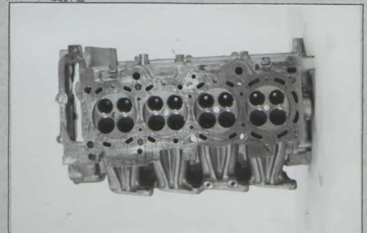
Culasse nue vue de dessous Bare cylinder head seen from below シリンダヘッド 単品下面
