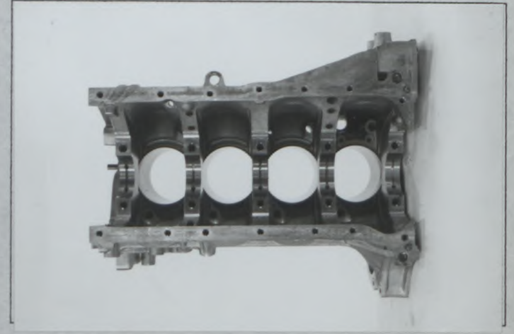
Profil gauche du bloc nu Left hand view of bare block シリンダブロック単品左側面
