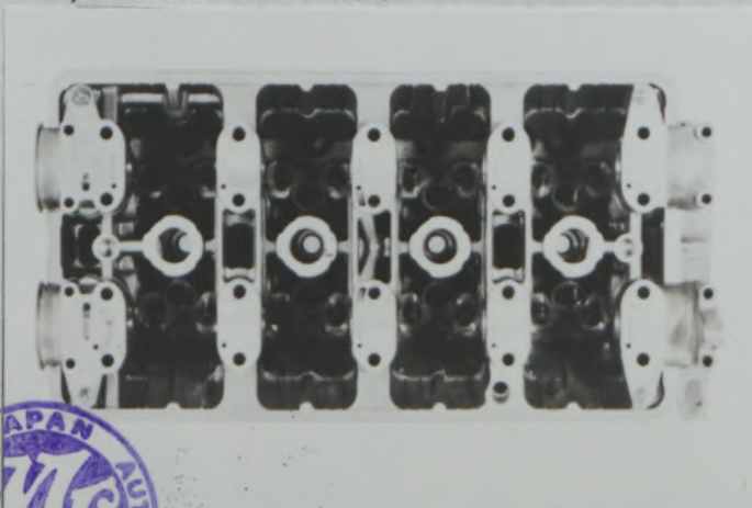
Culasse nue vue de dessus
