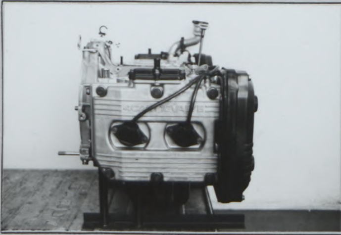
Profil droit du moteur complet déposé Right hand view of complete dismantled engine
