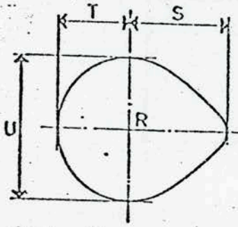
R 1 = Centro albero ad eccentrici.
